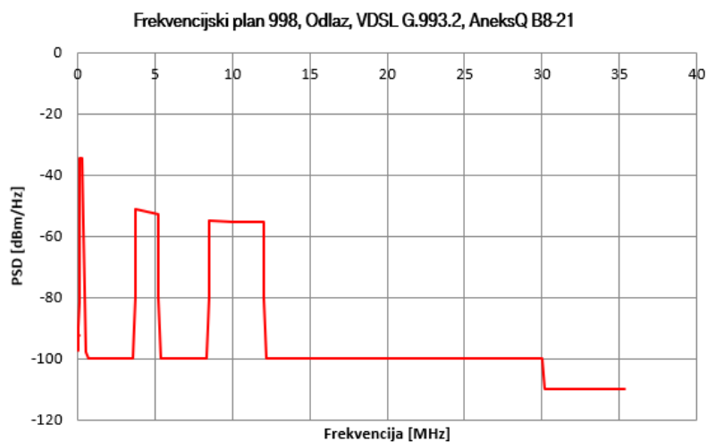
Slika 5.7.4 Frekvijski predložak za odlazni smjer prijenosa za VDSL2, frekvijski plan 998, B8-21
