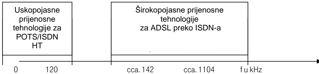
Slika 1. Frekventijski opseg za uskopolasne i širokopolasne prijenosne tehnologije
