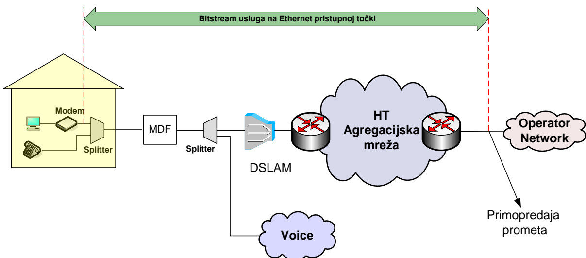
Slika 14. Veleprodajni širokopoljasi pristup za pružanje VoIP usluge na Ethernet razini u slučaju kada krajnji korisnik ostvaruje Osnovni pristup mreži putem usluge HT-a
