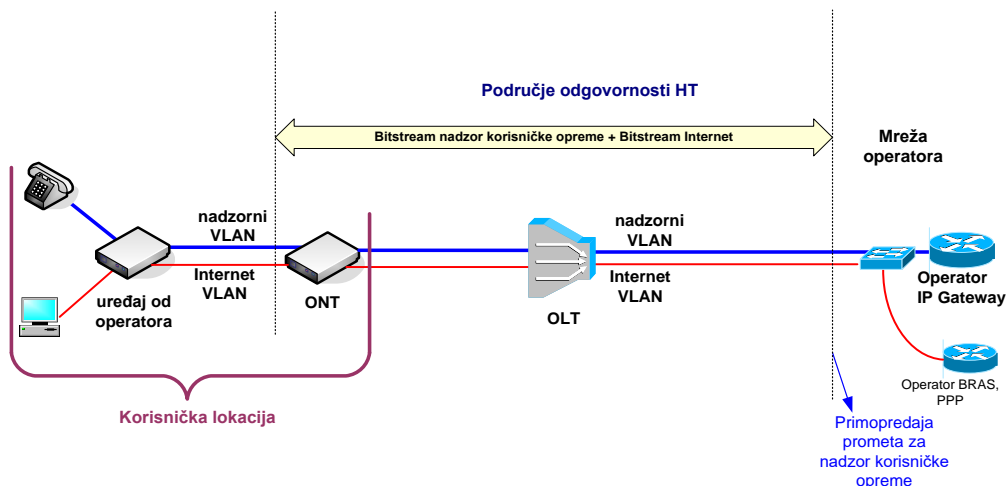
Slika 28. Veleprodajni širokopojsni pristup za pružanje usluge nadzora korisničke opreme preko FTTH pristupa (GPON) na OLT razini
