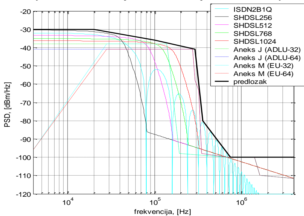
Slika 5.7.6 Frekvencijski predložak za odlazni smjer prijennosa (duge pretplatničke linije) za ADSL preko ISDN (aneks B).
