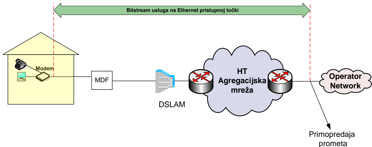
Slika 14. Veleprodajni širokopojasni pristup za pružanje VoIP usluge na Ethernet razini u slučaju kada krajnji korisnik ostvaruje Osnovni pristup mreži putem usluge HT-a
