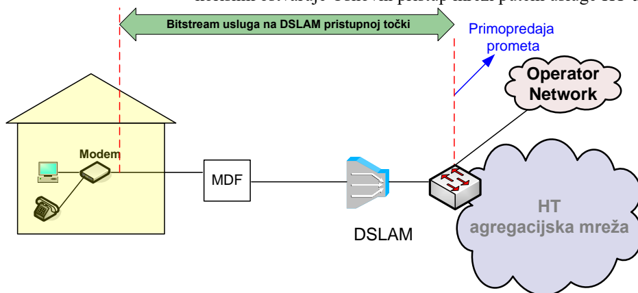
Slika 7. Veleprodajni širokopoljasni pristup za pružanje Internet usluge na DSLAM razini u slučaju kada krajnji korisnik ostvaruje Osnovni pristup mreži putem usluge HT-a
