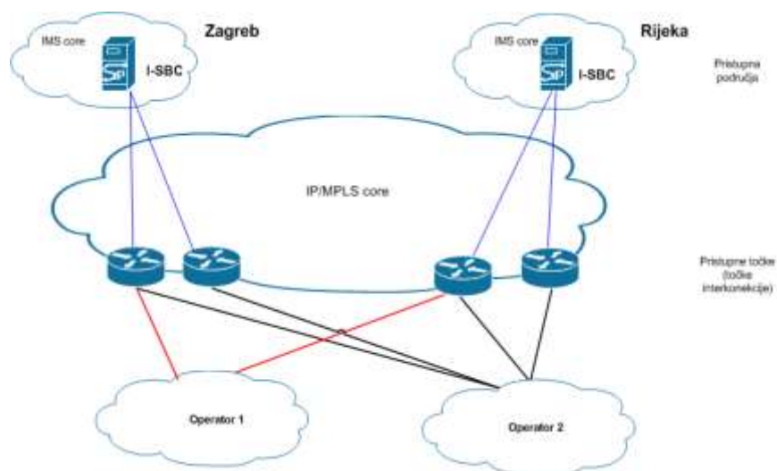
Slika 1. Arhitektura SIP međupovezivanja s HT mrežom
