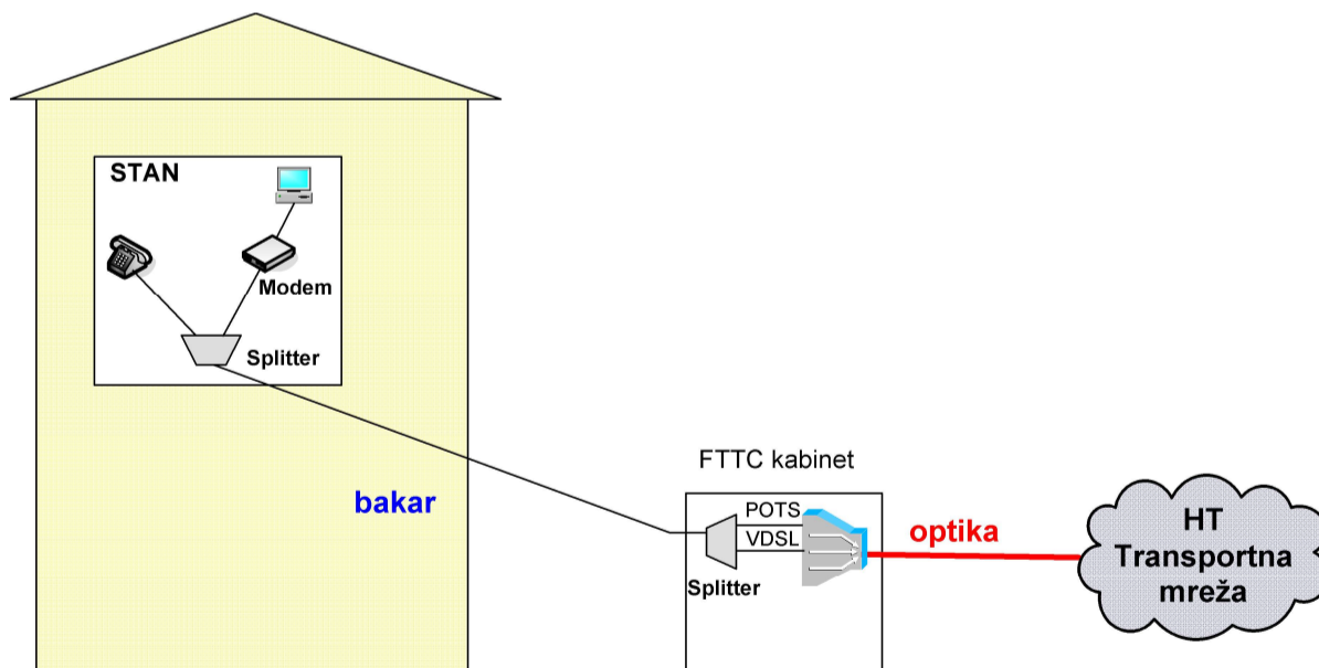
Slika 30. Način realizacije FTTC koncepta u pristupnoj mreži
