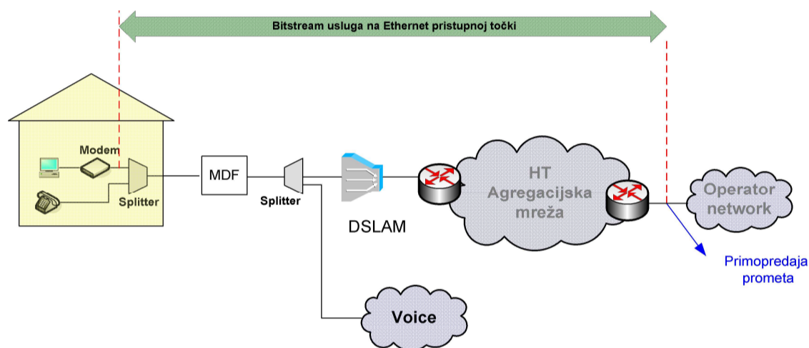
Slika 3. Veleprodajni širokopojsni pristup za pružanje Internet usluge na Ethernet razini u slučaju kada Krajnji korisnik ostvaruje Osnovni pristup mreži putem usluge HT-a.
