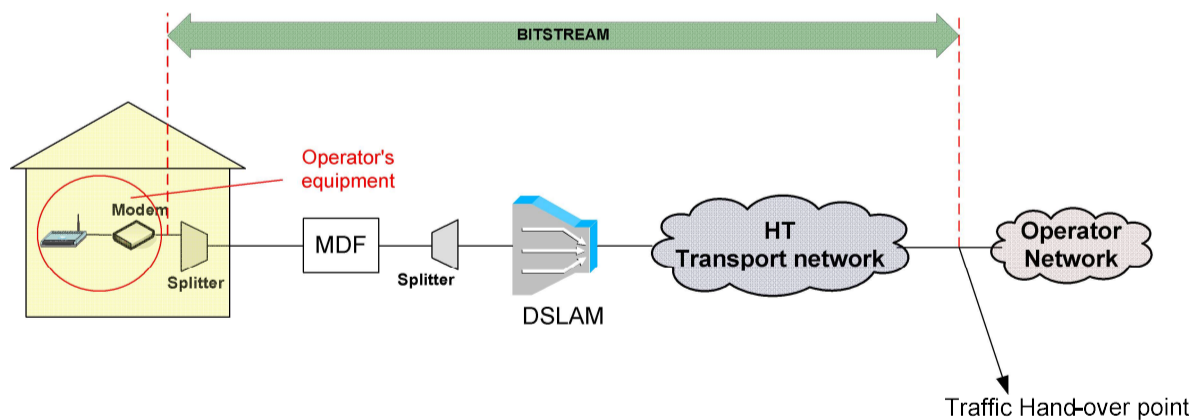
Slika 32. Koncept posebnog virtualnog kanala za Podatkovnu uslugu
