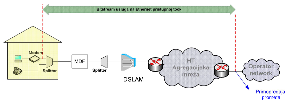
Slika 3. Veleprodajni širokopojsni pristup za pružanje Internet usluge na Ethernet razini u slučaju kada Krajnji korisnik ostvaruje Osnovni pristup mreži putem usluge HT-a.
