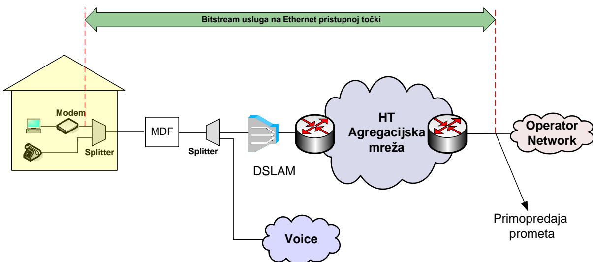
Slika 14. Veleprodajni širokopolasni pristup za pružanje VoIP usluge na Ethernet razini u slučaju kada krajnji korisnik ostvaruje Osnovni pristup mreži putem usluge HT-a
