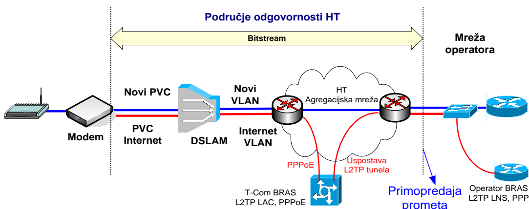
Slika 33. Realizacija posebnog virtualnog kanala za Podatkovnu uslugu preko ADSL pristupa
