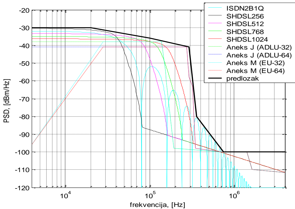
Slika 5.7.6 Frekvencijski predložak za odlazni smjer prijena (duge pretplatničke linije) za ADSL preko ISDN (aneks B).
