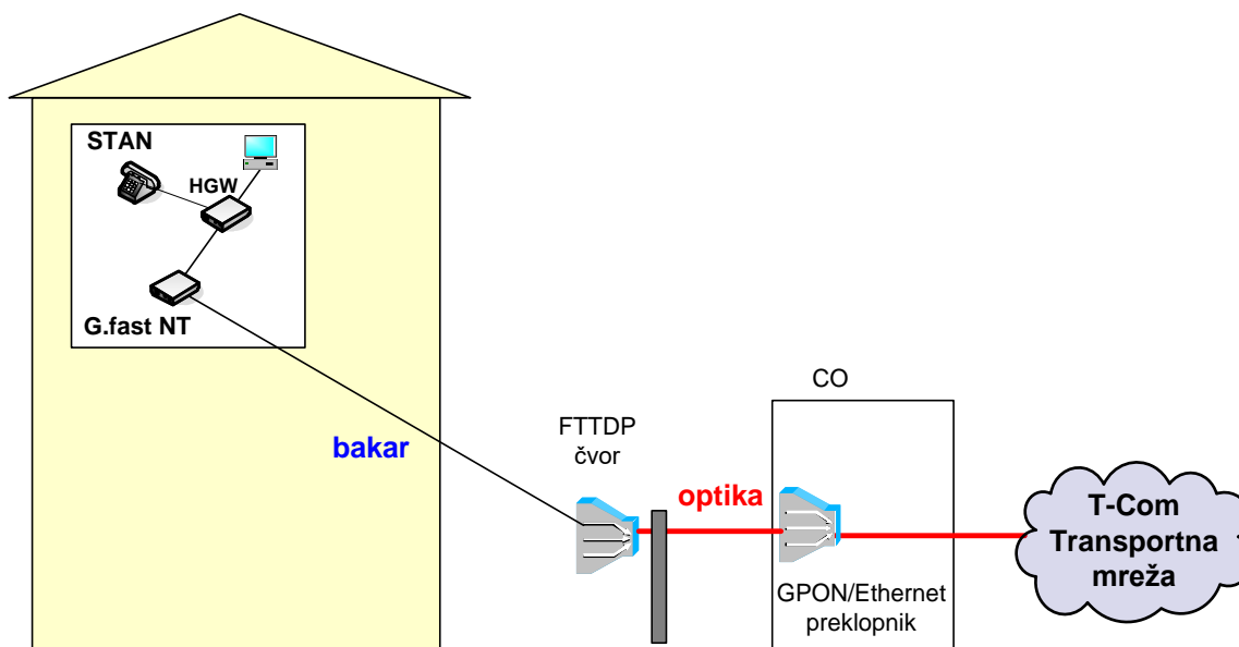
Slika 36a. Način realizacije FTTH koncepta sa G.fast tehnologijom u pristupnoj mreži
